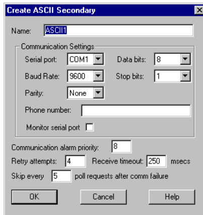
Figure 3-9. ASCII Definition Parameters Dialog Box
